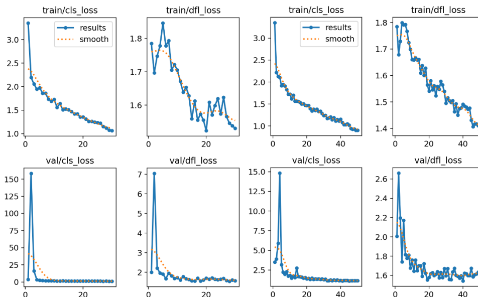
Abb. 8: Ergebnisse von YOLOv8m in 30 Epochen (links) und 50 Epochen (rechts)
