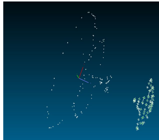
Abb. 6: Geplante (links) und tatsächlich geflogene Aufnahme­konfiguration für eine Elevationsposition
