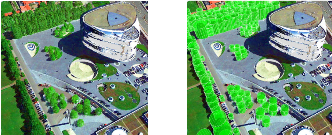
Abb. 5: Darstellung der integrierten Ergebnisse des gesamten M3D-Datensatzes ( links : kolorierte Punktwolke als Eingabedaten, rechts : durch Datenintegration rekonstruierte gemittelte Zylinder)
