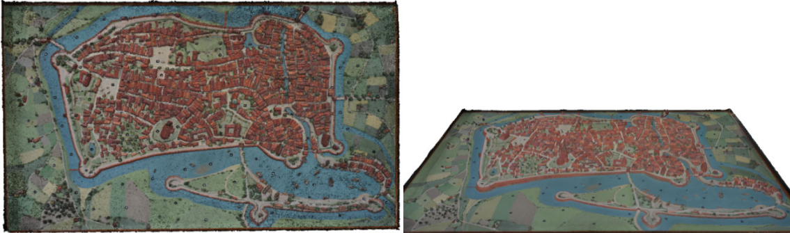
Abb. 3: Dichte 3D-Punktwolke des physikalischen Stadtmodells von Stade im Jahr 1620 (links) und perspektivische Ansicht des texturierten, vermaschten 3D-Modells (rechts)
