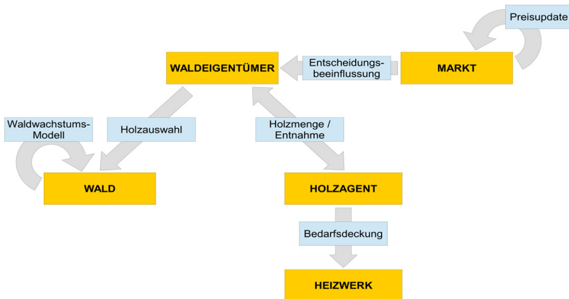
Abb. 1: Aufbau und Zusammenspiel der Modellkomponenten
