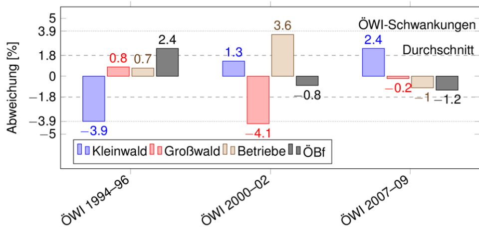
Abb. 2: Ergebnisse der Validierung. Prozentuale Abweichung der Entnahmemengen pro Eigentumsklasse im Modell bezogen auf die im Zuge der ÖWI erhobenen Entnahmemengen
