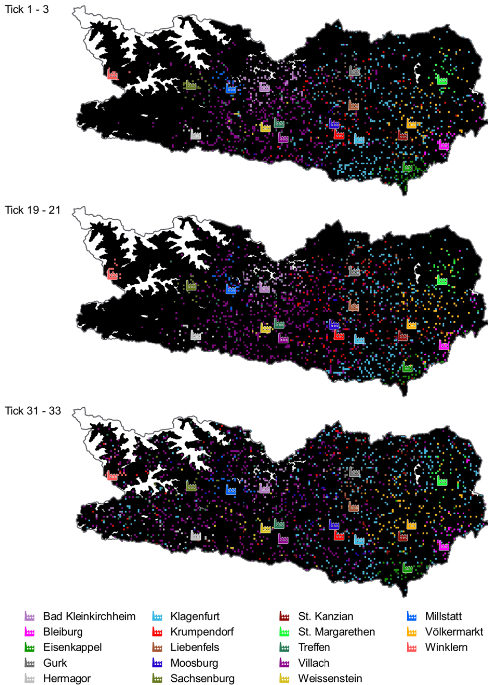
Abb. 4: Raumzeitliche Entwicklung der Holzentnahmebereiche der Heizwerke. Mit knapper werdendem Holzvorrat verschieben sich die Entnahmebereich von lokal um die Standorte immer weiter in periphere Bereiche.
