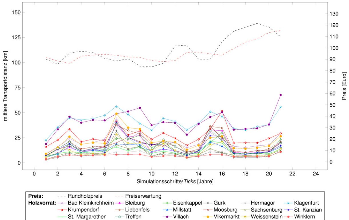
Abb. 3: Entwicklung der mittleren Transportdistanz zu den Heizwerken pro Holzbeschaffung über den Simulationsverlauf von 21 Jahren. Dieser ist im Bezug zur extrapolierten Holzpreisentwicklung und der mittleren Preiserwartung der Waldeigentümer dargestellt. Liegt die Erwartung unter dem Preis müssen weniger Transportkosten in Kauf genommen werden und umgekehrt.
